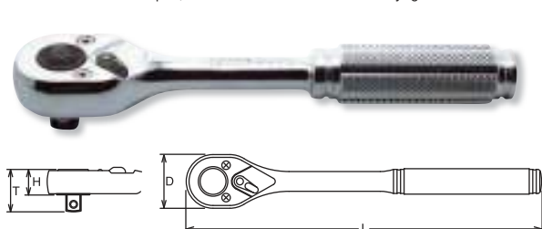
2753NB Reversible Ratchet with quick release button Knarre, verstellbar mit Entriegelungsknopf Cliquet, réversible avec bouton de débrayage
